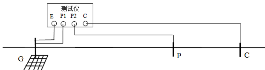
G — 被试接地装置 C — 电流极 P — 电位
