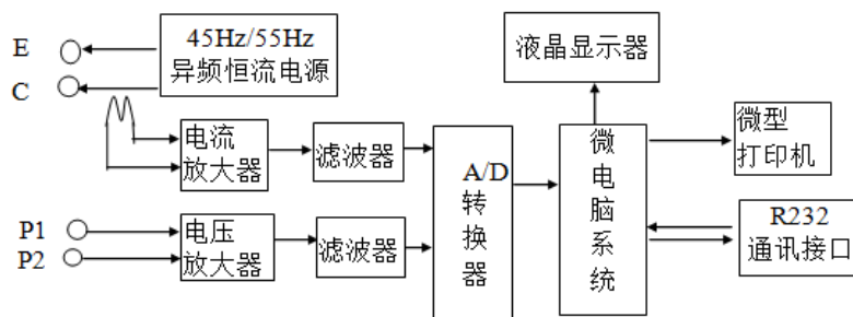
图 1 仪器内部结构图
