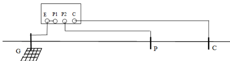
G — 被试接地装置 C — 电流极 P — 电位
