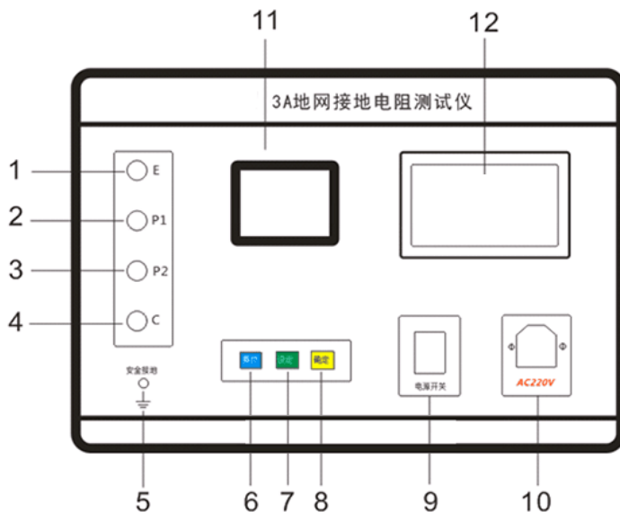
仪器面板布置图
