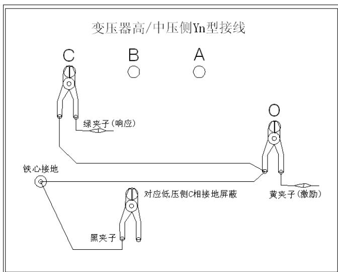
Yn 形测量 C 相接线示意图
