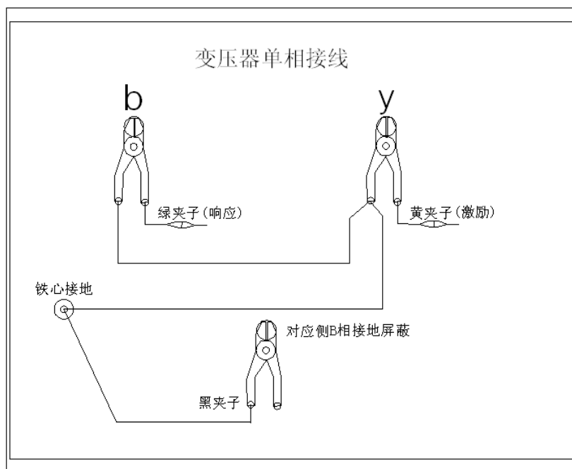
b-y 测量接线示意图
