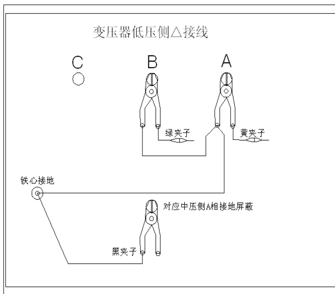
\Delta 形测量 A 相接线示意图
