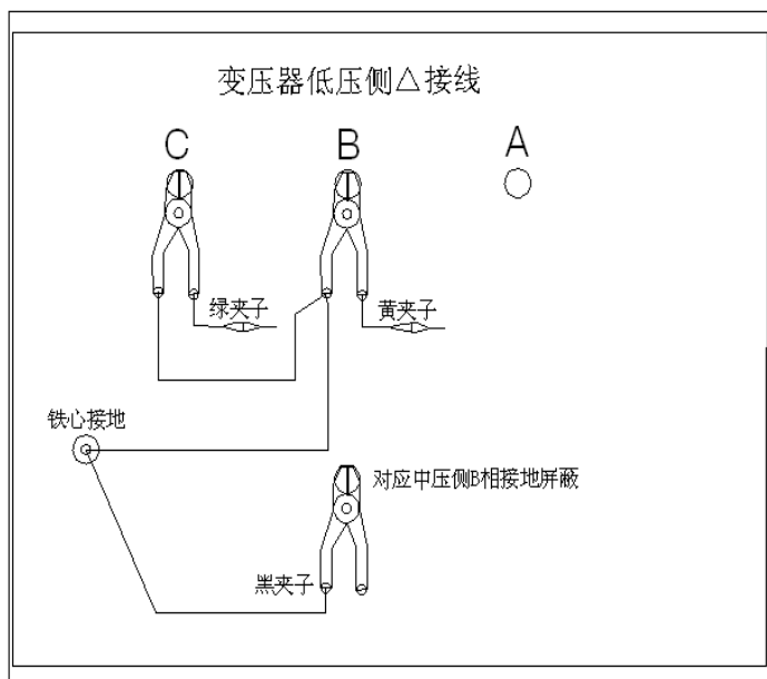
\Delta 形测量 B 相接线示意图
