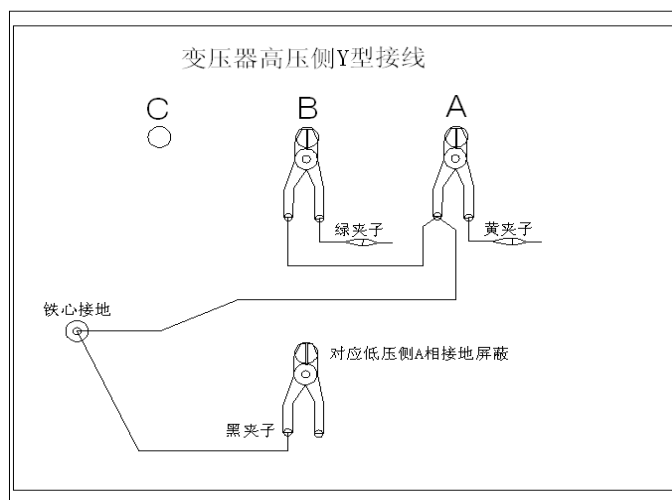
Y 形测量 A 相接线示意图
