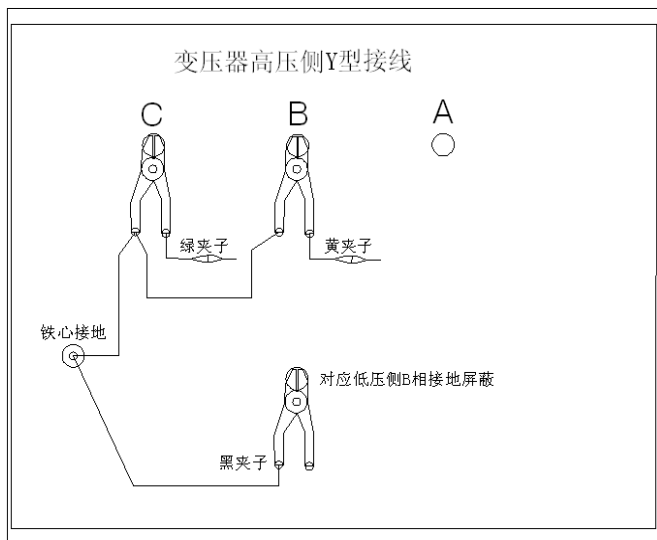
Y形测量 B 相接线示意图
