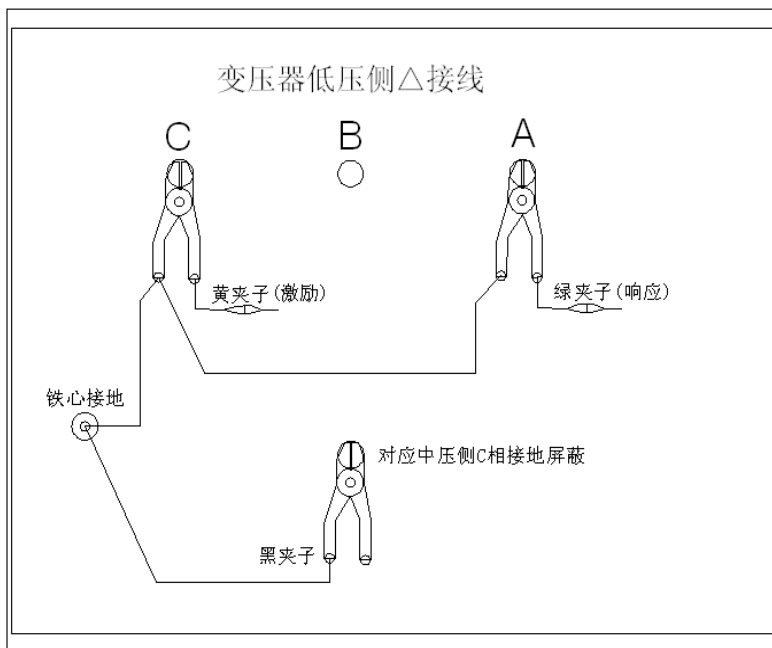
△形测量 C 相接线示意图
