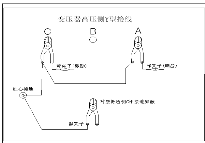
Y形测量 C 相接线示意图
