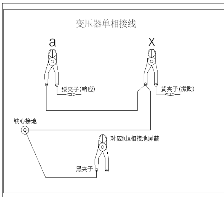
a-x 测量接线示意图
