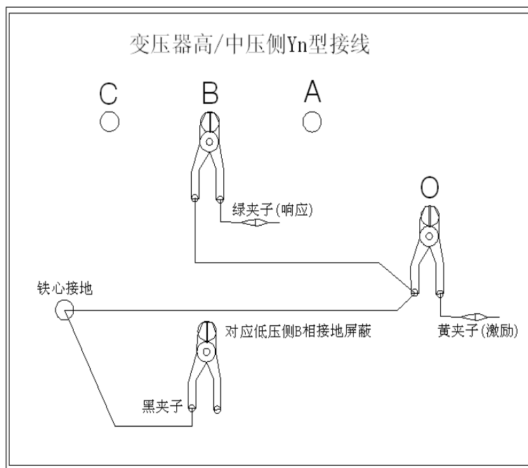
Yn 形测量 B 相接线示意图
