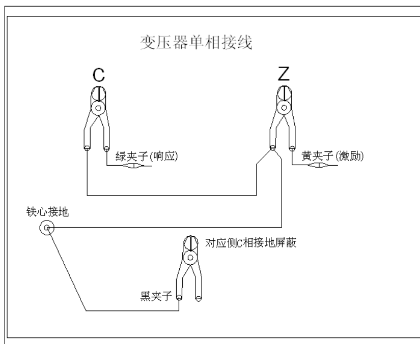
c-z 测量接线示意图
