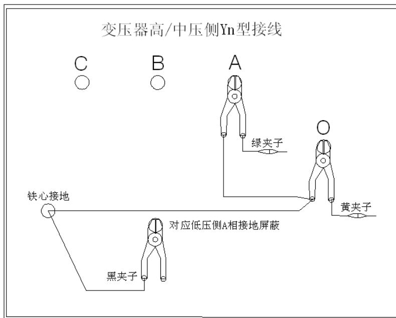
Yn 形测量 A 相接线示意图
